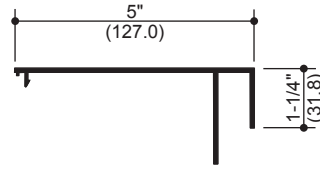
069266 5" STOOL TRIM
